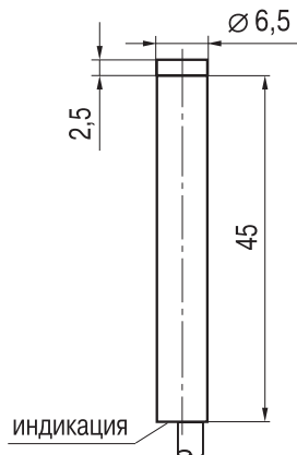
Габаритный чертёж
